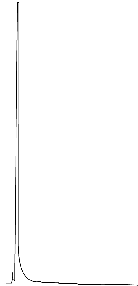
图 A.1 丁酸乙酯典型气相色谱图(面积归一化法)
